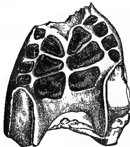
PLACODUS GIGAS. Crushing Teeth. ( Trias. )
